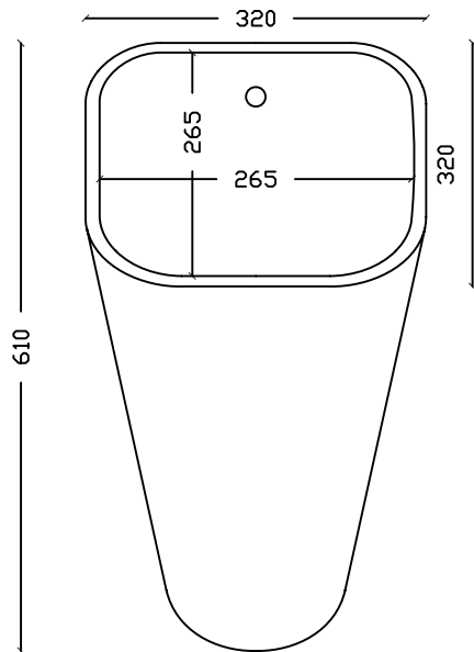
Vista frontale
