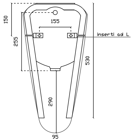
Vista posteriore
