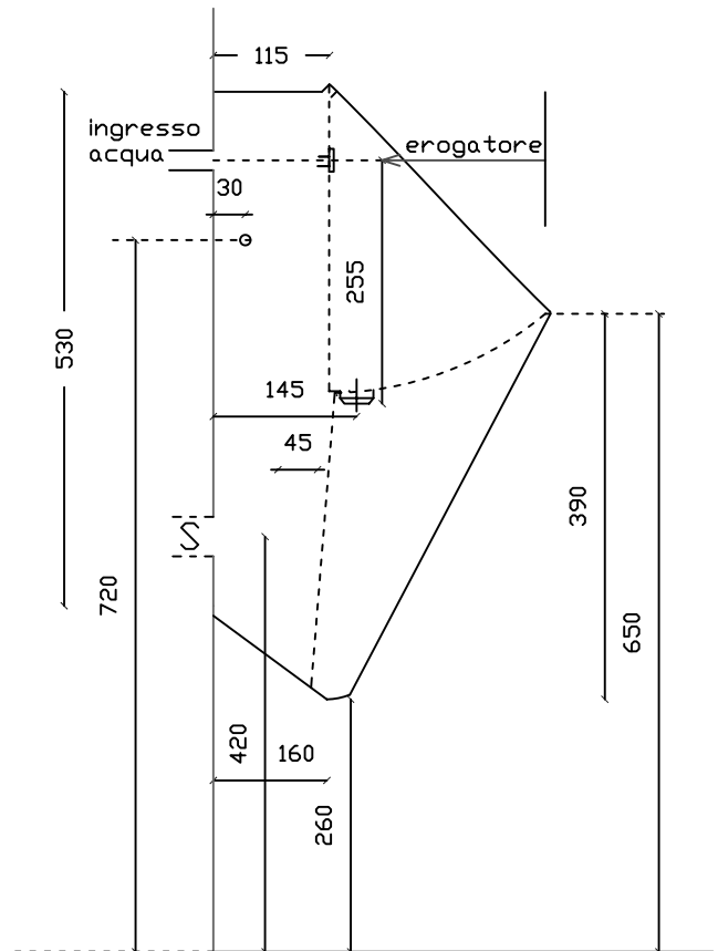
Vista laterale
