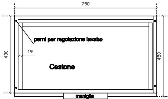
Vista dall'alto
