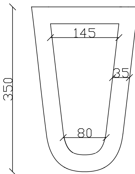
Vista posteriore
