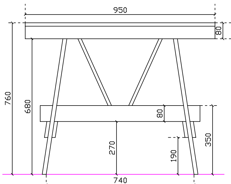
Vista frontale
